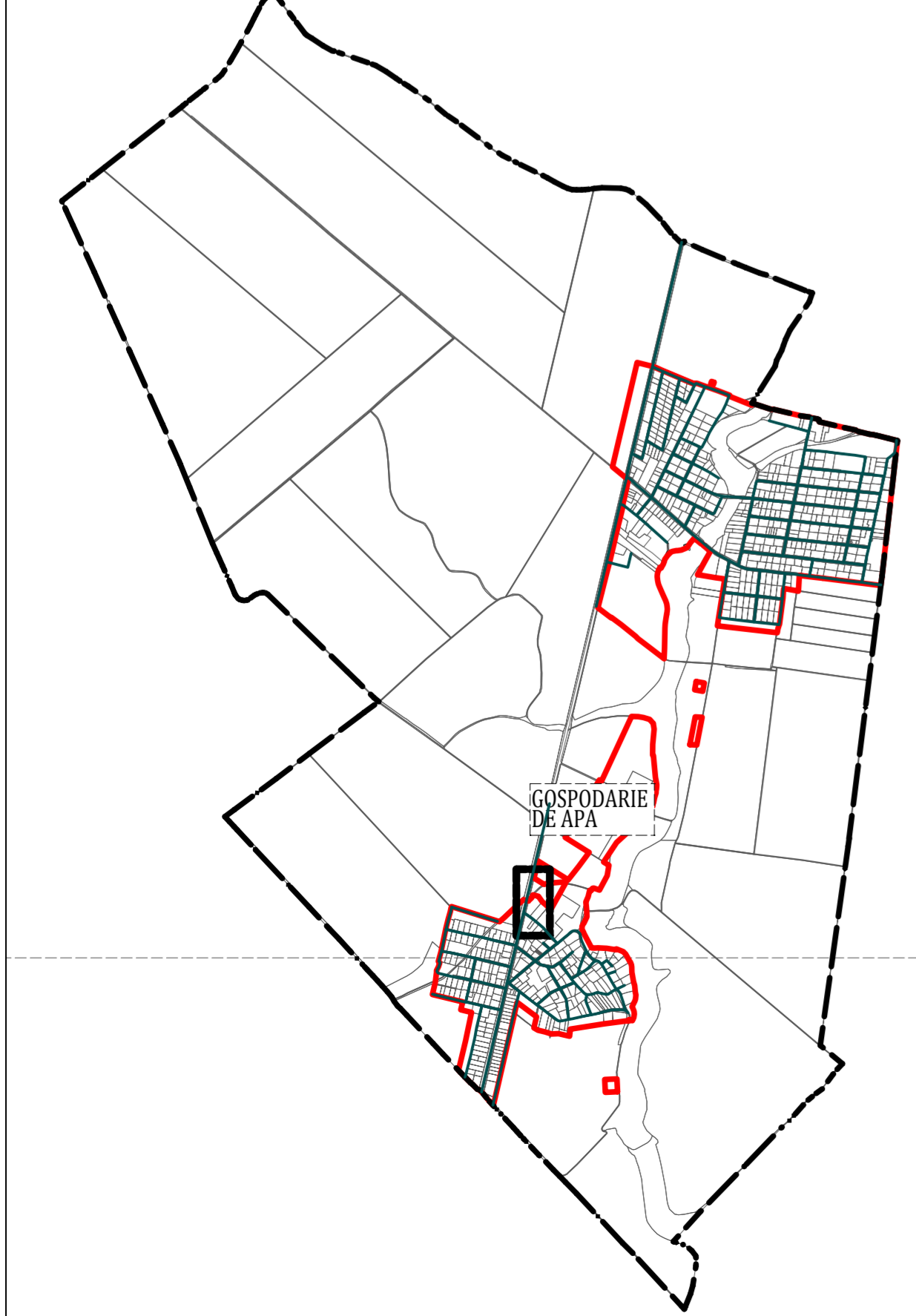
p1211 realizarea rețelei de alimentare cu apă
